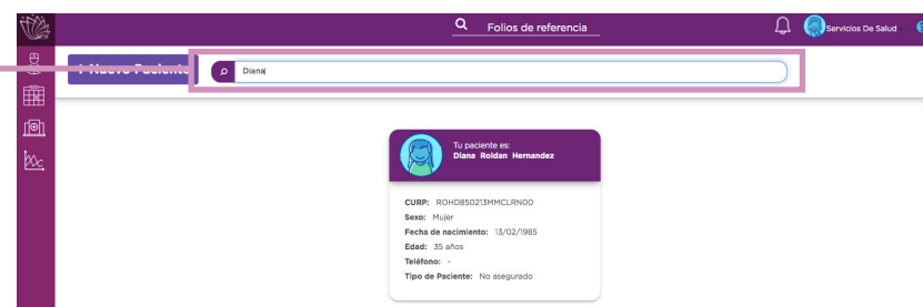
Figura 5: Búsqueda paciente
