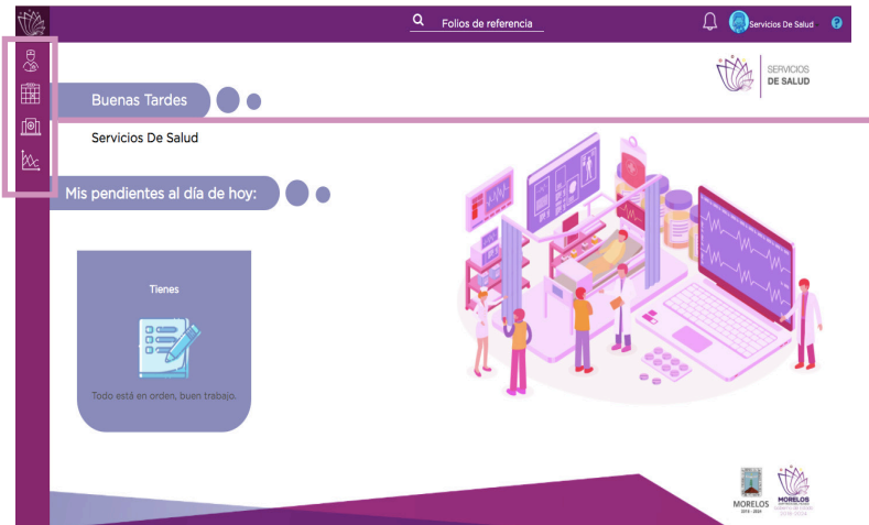
Figura 3: Pantalla inicial
