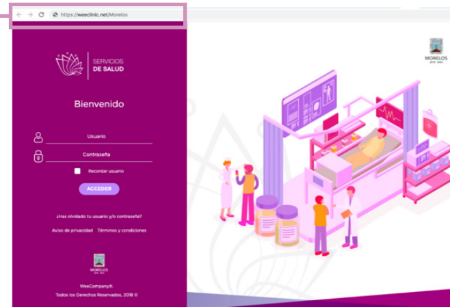
Figura 1: Plataforma sirce
