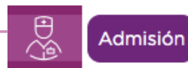
Figura 4: Módulo Admisión
